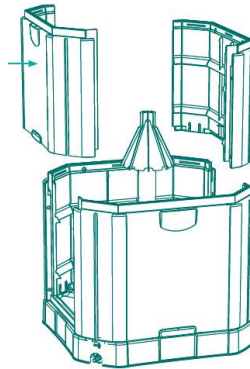
Külgpaneelide konksud
